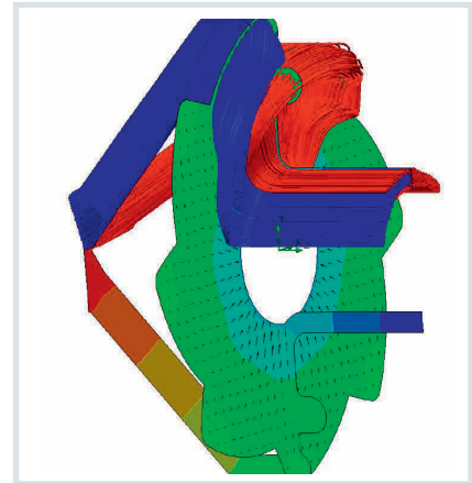
Bild 1. Prinzip der Zirkularverteilung; links ein Zirkularverteiler, rechts die Simulation der radialen Umfangsverteilung nach der Schmelzevorverteilung (© ETA)
