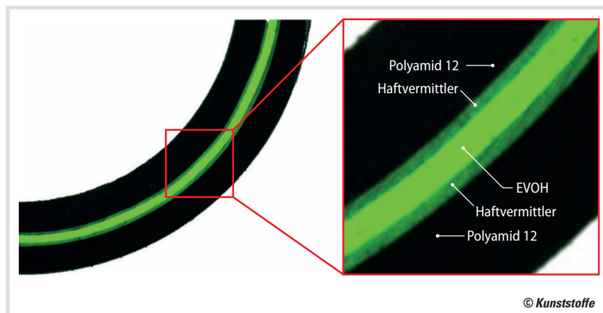
Bild 2. 5-schichtige Kraftstoffleitung; Links der Rohrquerschnitt, rechts eine Detailsicht (Quelle: ETA)
